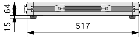
正面図
